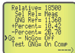
Finestre di impostazione dei parametri riguardanti la misura relativa, il test Go - No Go e la compensazione della misura in base alla temperatura ambiente e di riferimento.
