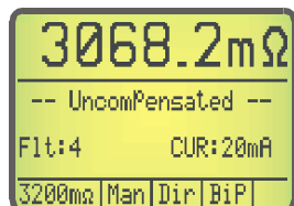
Misura principale sulla portata di 3200mΩ, in modalità misura bipolare.
