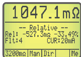
Misura principale + misura relativa assoluta e percentuale.
