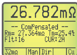
Misura compensata + misura alla temperatura ambiente e indicazione della temperatura ambiente impostata/misurata.
