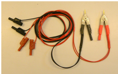
Coppia cavetti KELVIN - cavo L=1,60mt - pinze con apertura max 7mm
